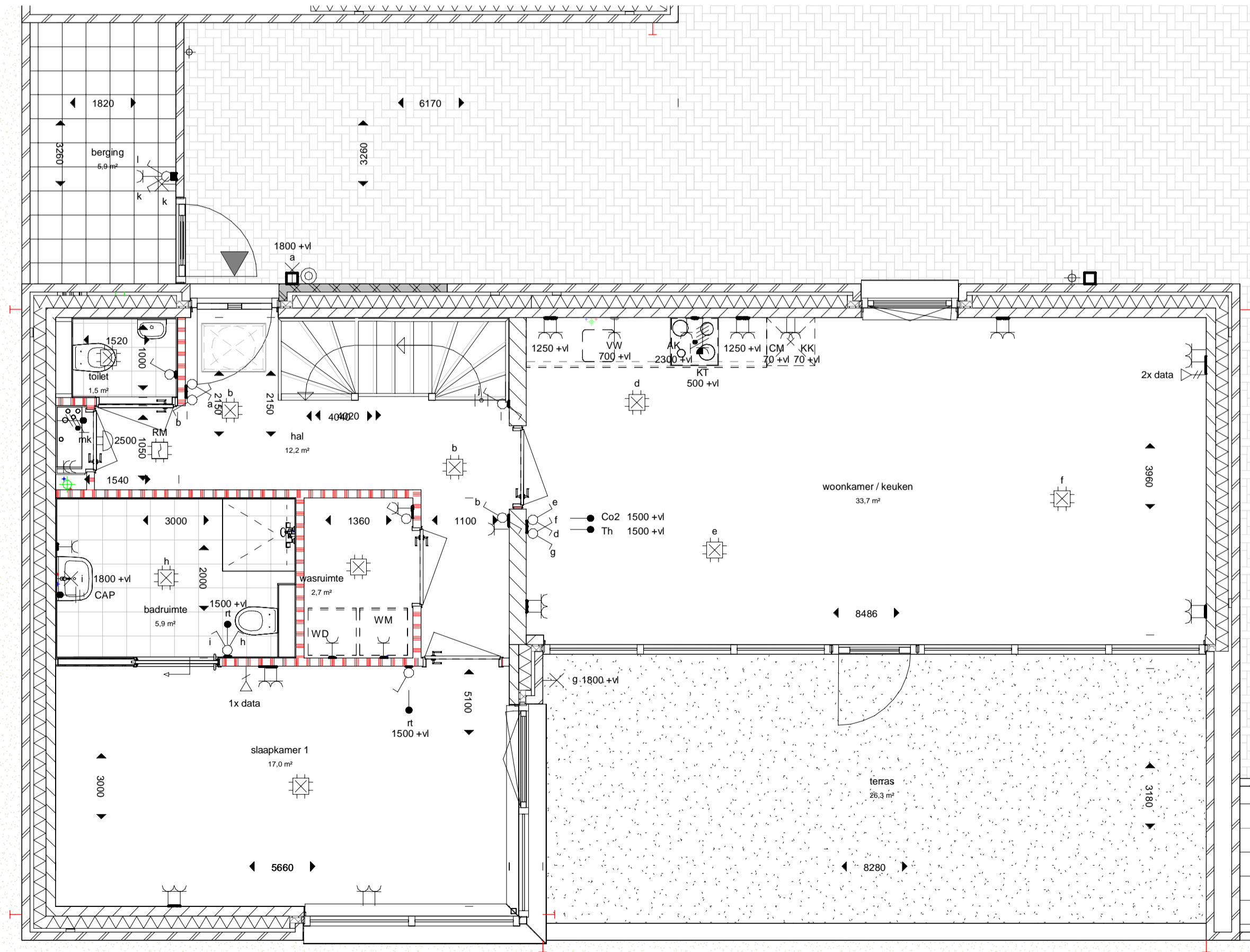
begane grond 1:50
