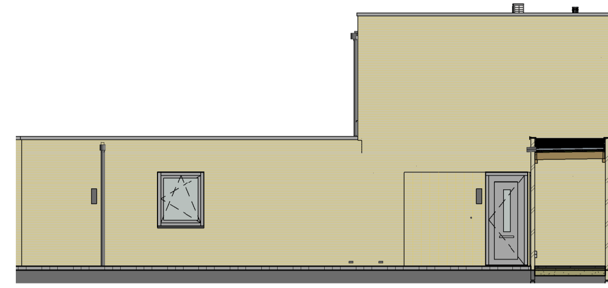
rechtegevel 1:100
