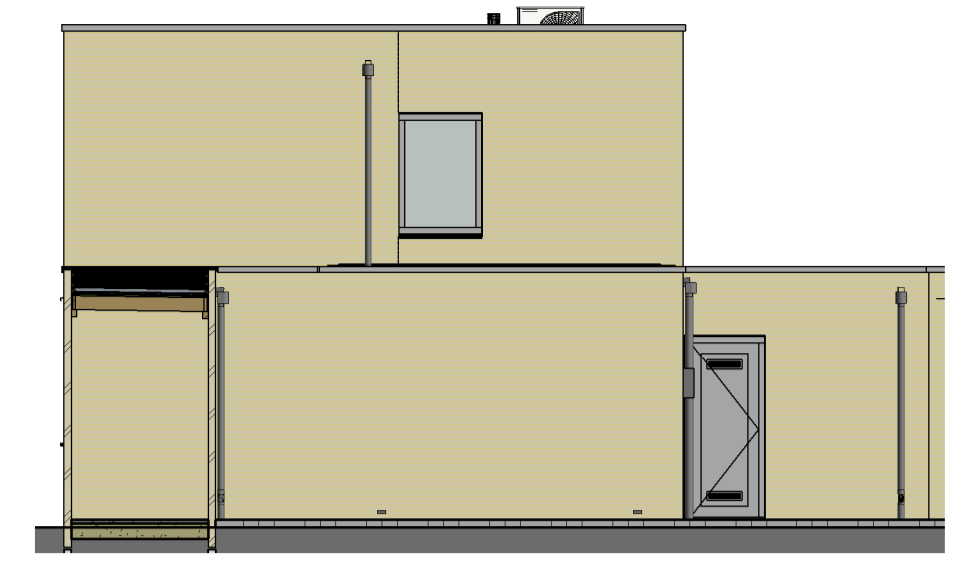
voorgevel 1:100
