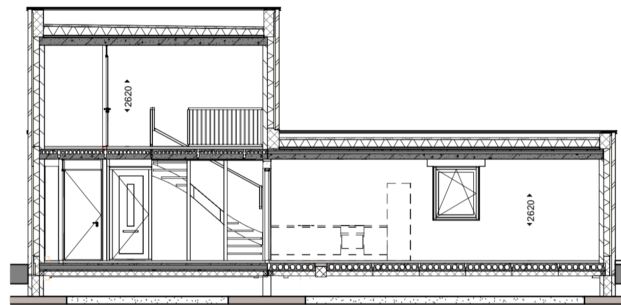
doorsnede 1:100
