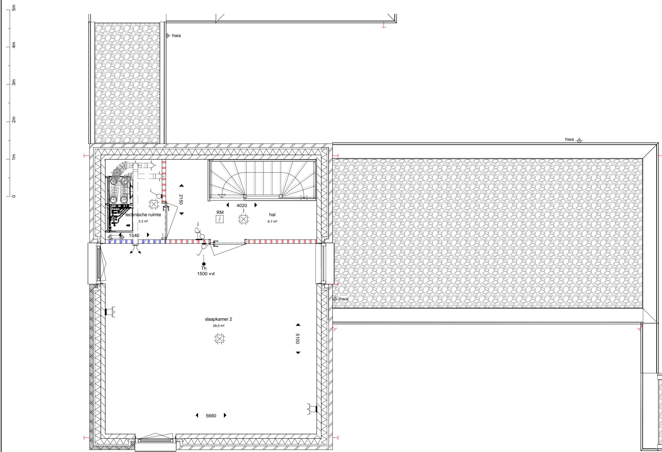
verdieping 1:50
