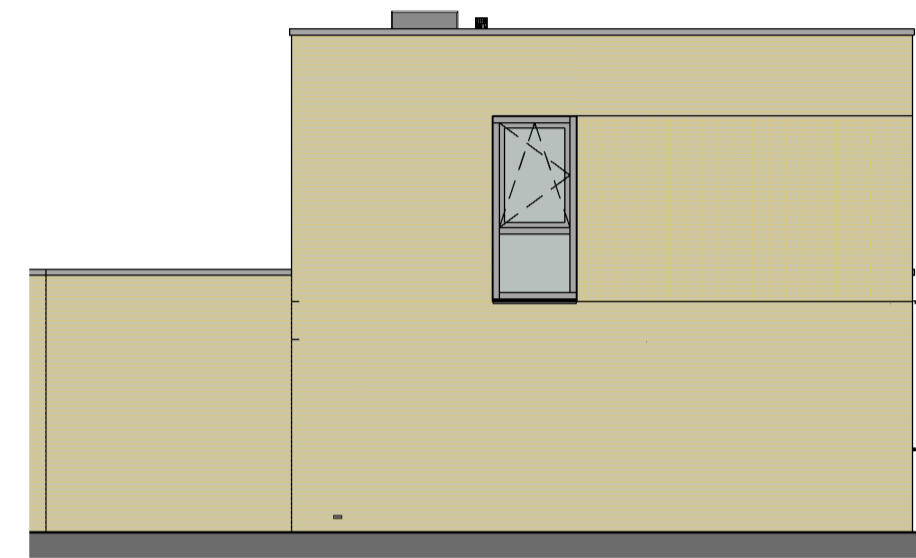
achtergevel 1:100
