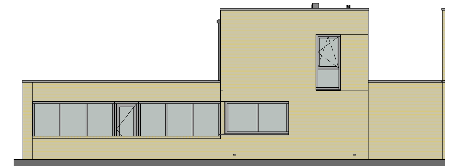
westgevel 1:100
