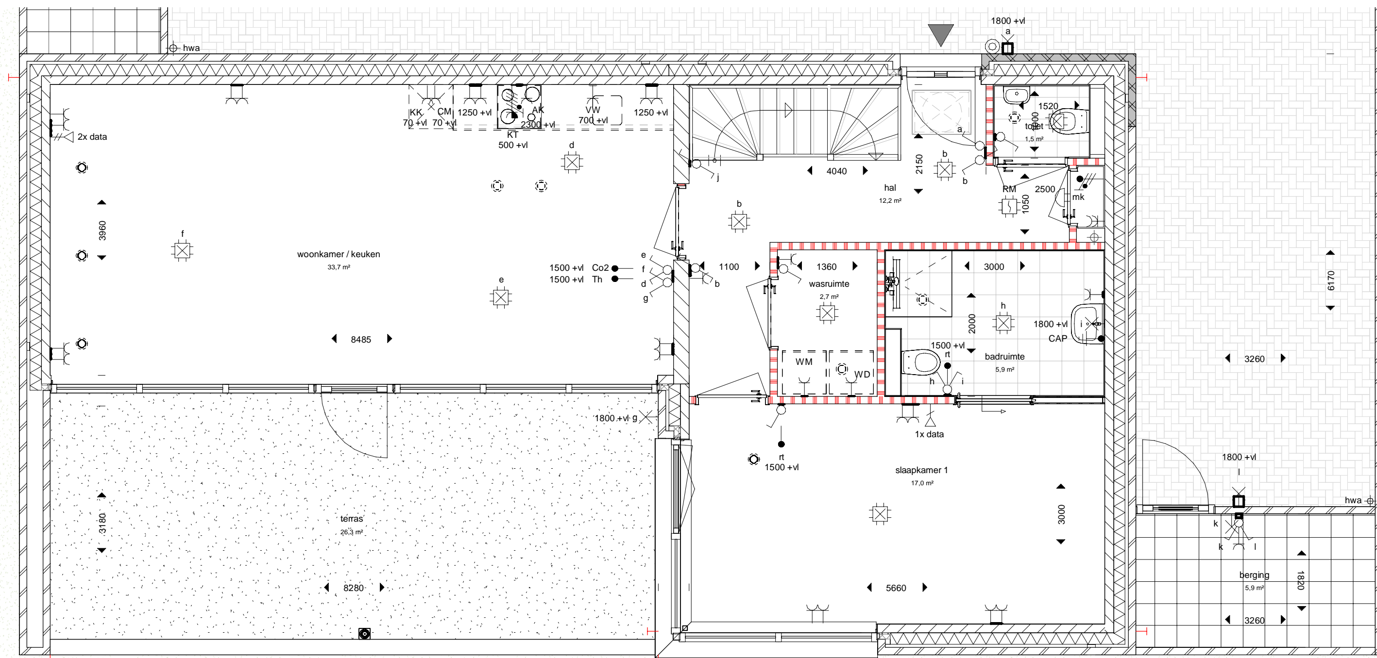
begane grond 1:50
