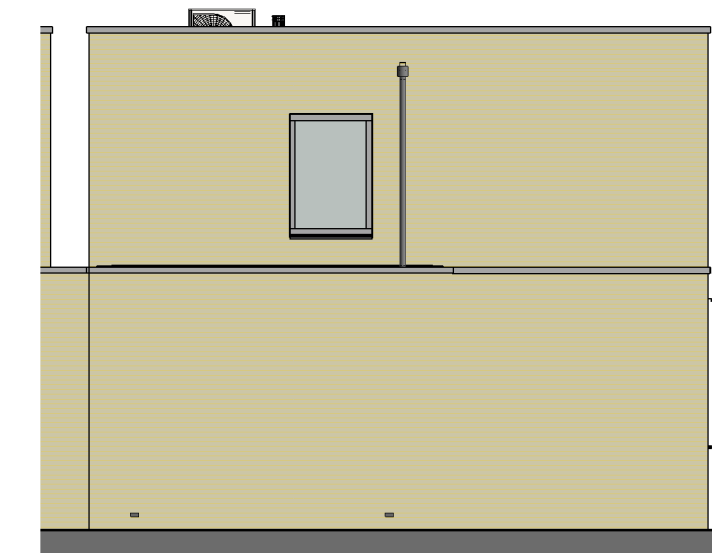
noordgevel 1:100
