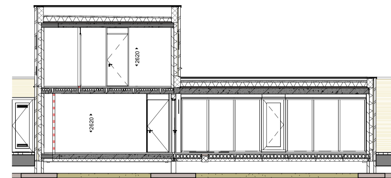
doorsnede 1:100
