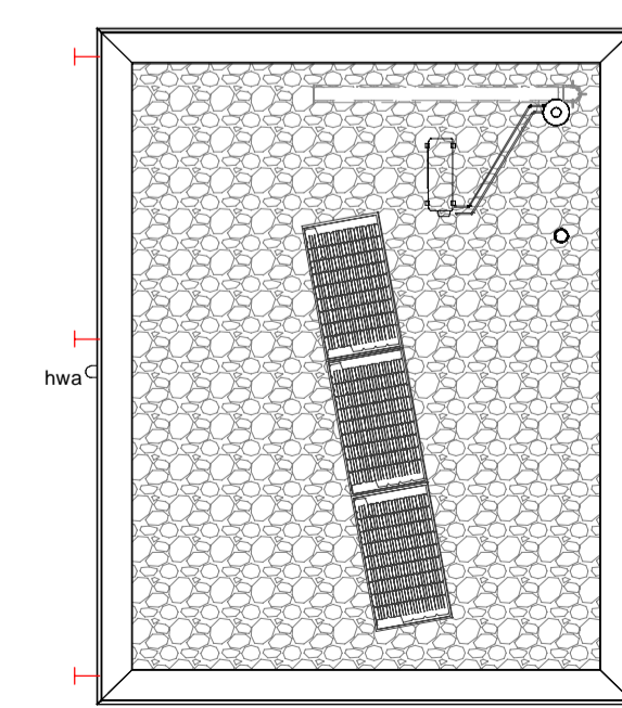
dak 1:100
